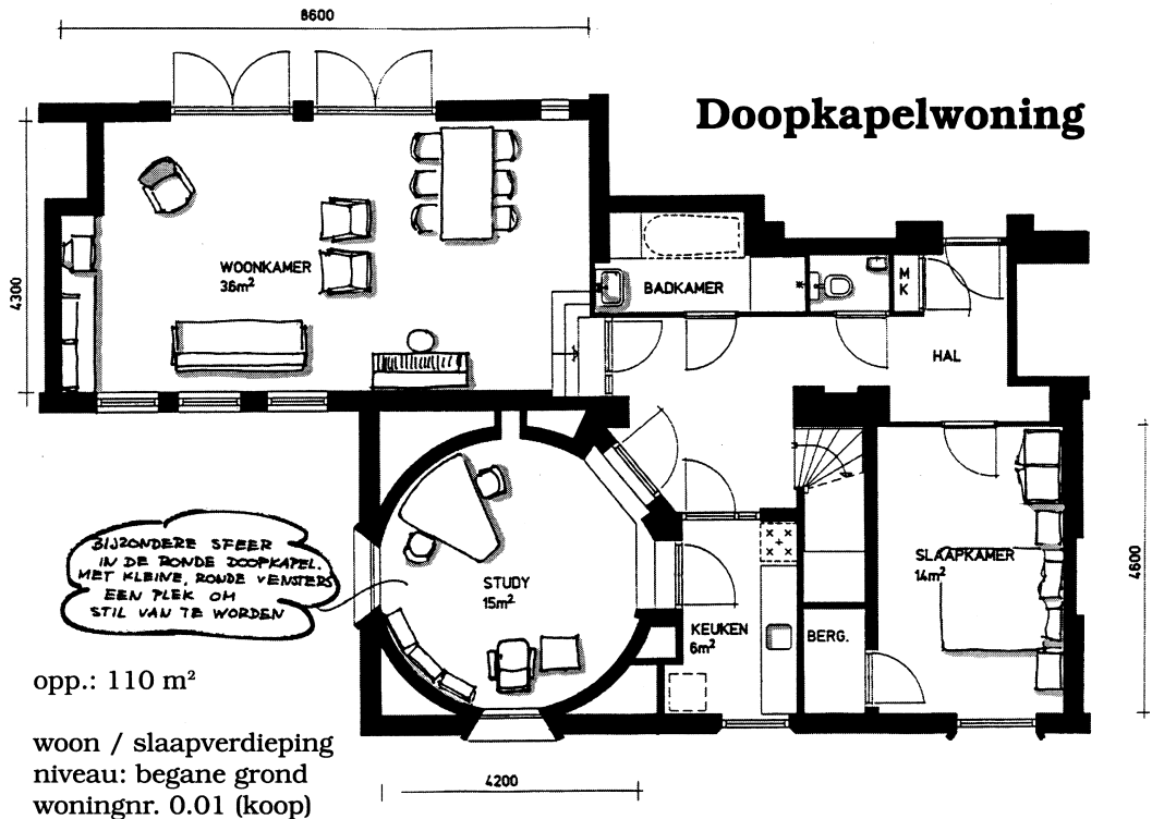
Plattegrond van de doopkapelwoning zoals afgebeeld in het boekje Wonen in de St. Josephkerk . De doopkapelwoning was één van de koopwoningen.
