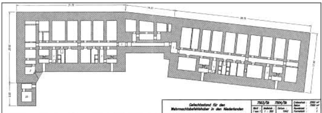
Plattegrond van de Blaskowitzbunker aan de Verdilaan. Duidelijk is te zien dat de bunker uit twee verschillende delen is opgebouwd. Bouwtekening uit 1943. Uit: De commandobunker van Hilversum.
