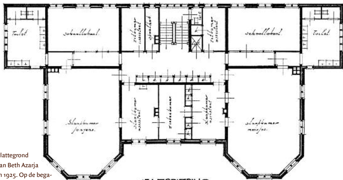
1E VERDIEPING.
