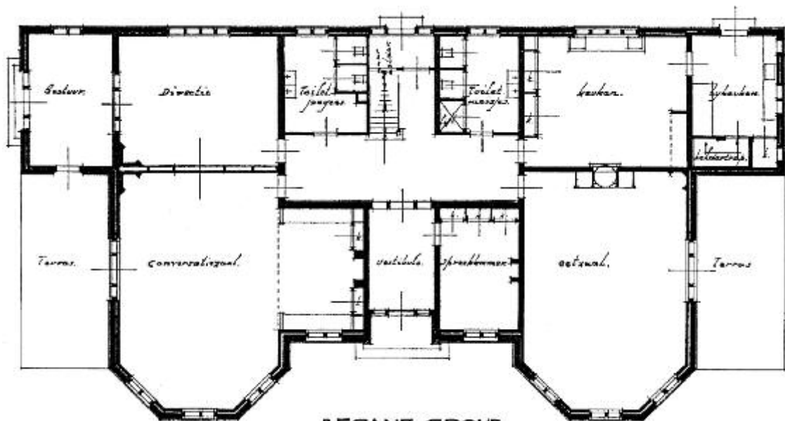
BEGANE GROND.
